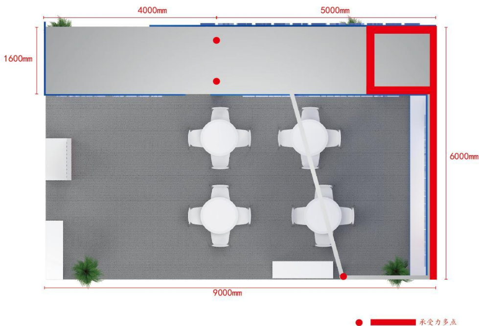
主体承受力结构图
